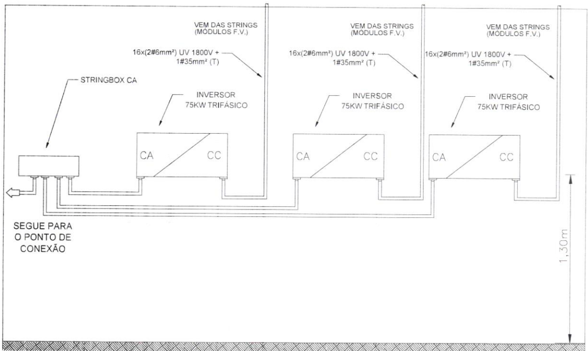
VISTA FRONTAL SEM ESCALA
