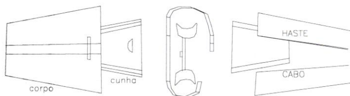
CONECTOR DE ATERRAMENTO
