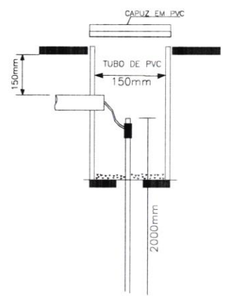
DETALHE DA CAIXA DE ATERRAMENTO
