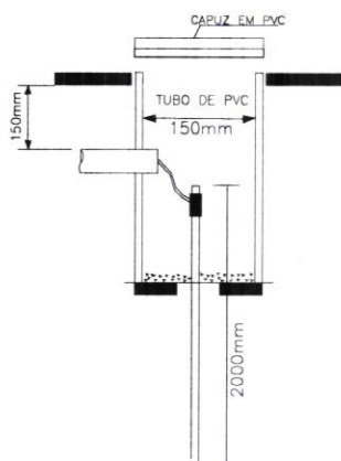
DETALHE DA CAIXA DE ATERRAMENTO
